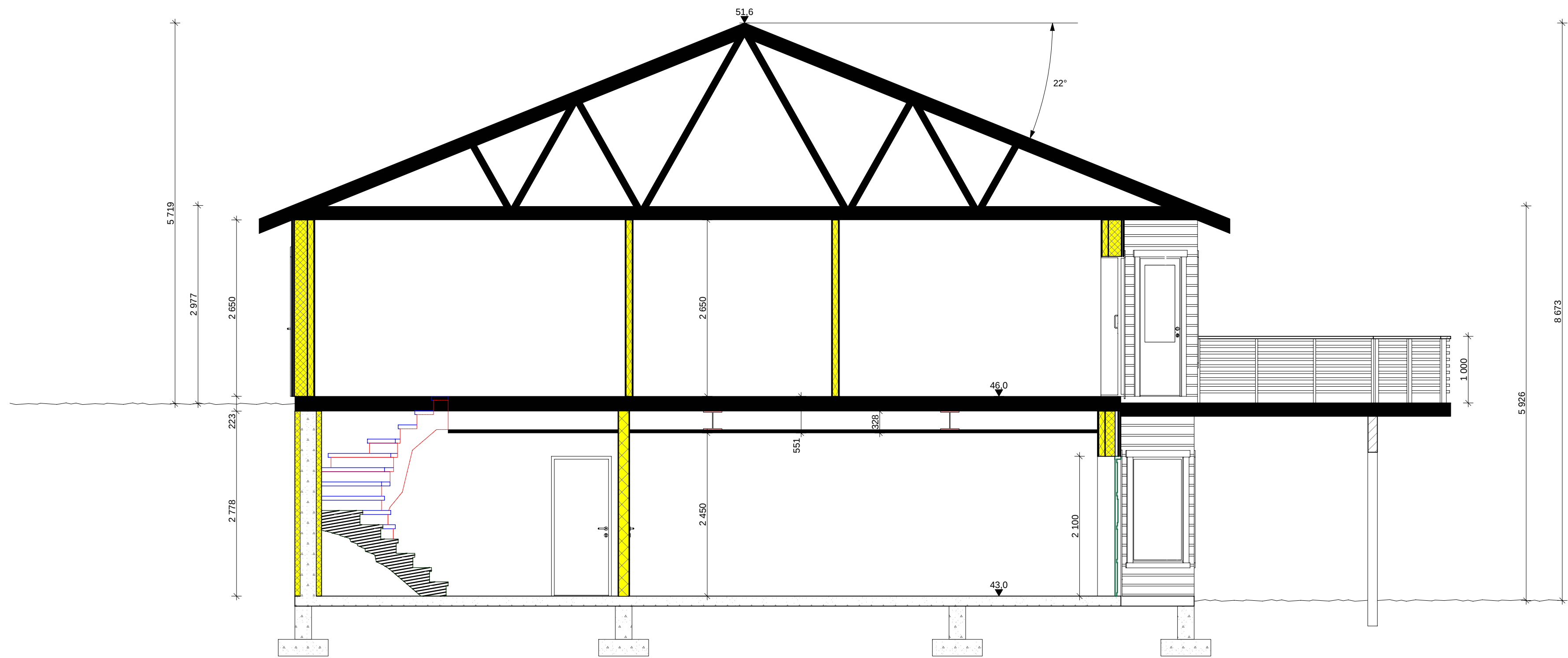
A - A 1:50
