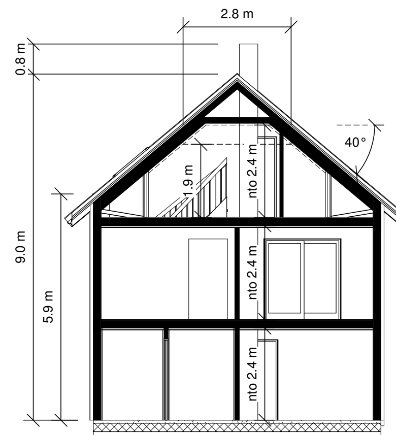
SNITT A-A
