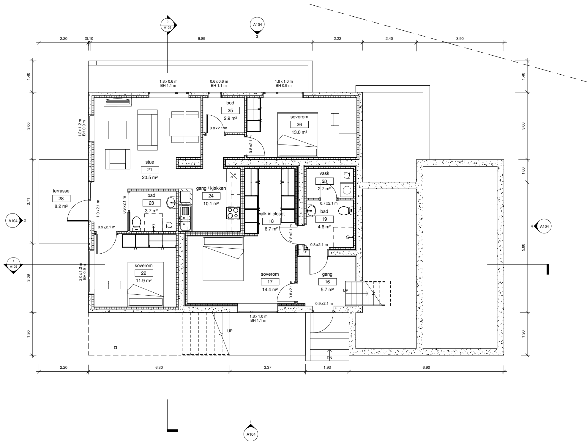
① KJELLERETASJE 1 : 50
