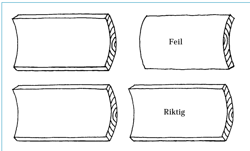
Figur 7. Det er viktig å skjote bord med lik årringretning. (Krumning er sterkt overdrevet.)
