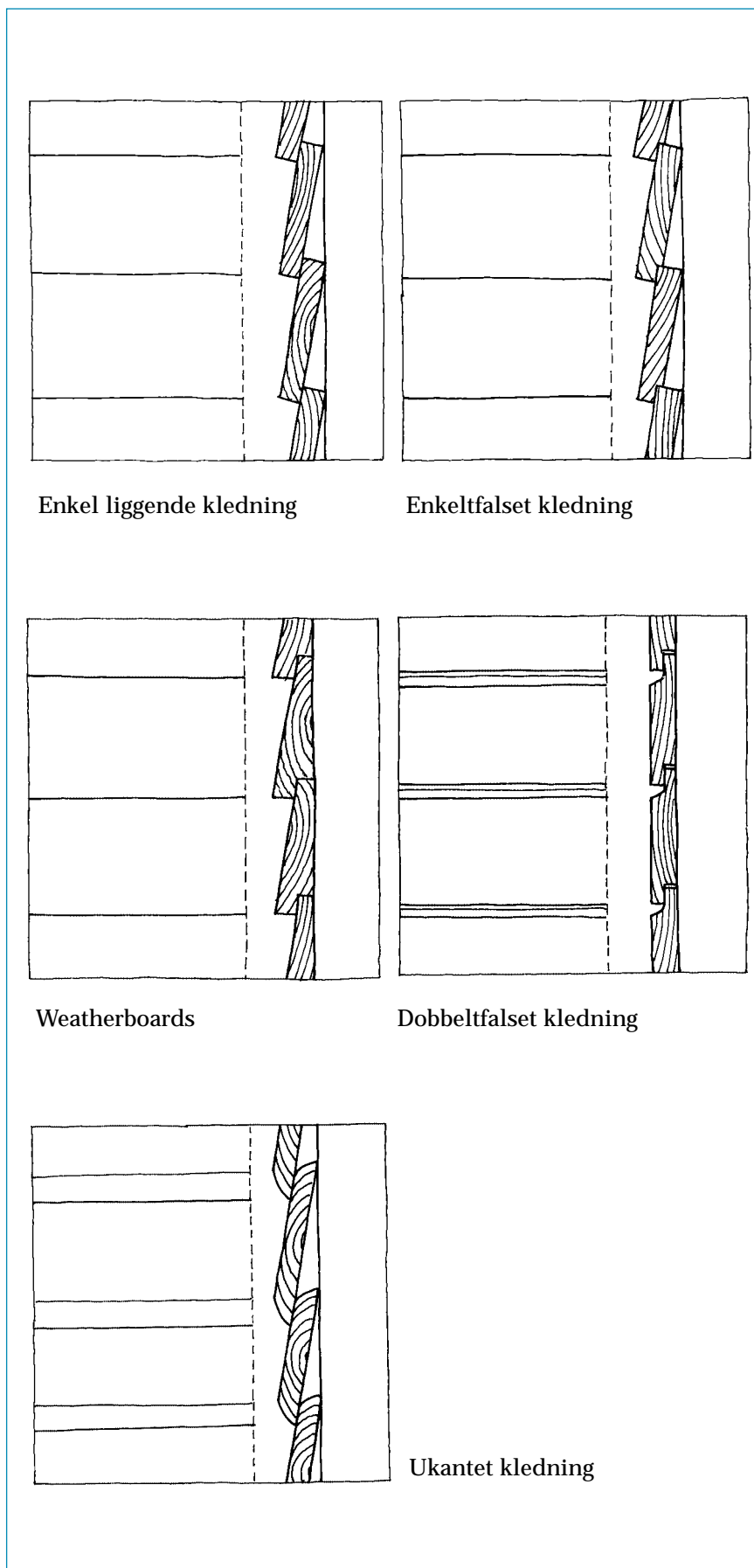
Fig. 4. Eksempel på liggende kledning.
