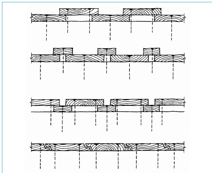
Fig 3. Riktig spikring av stående kledning.
