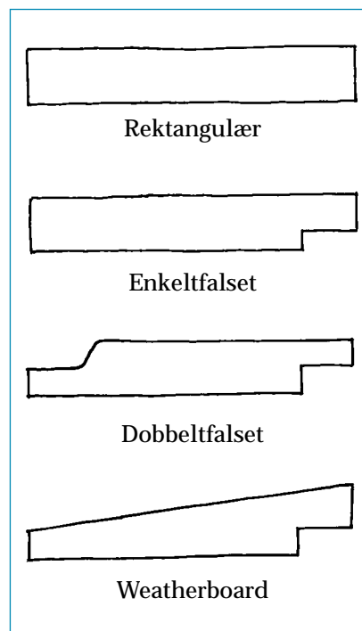
Fig 1. Standardiserte kledningsbord i NS 3186.
