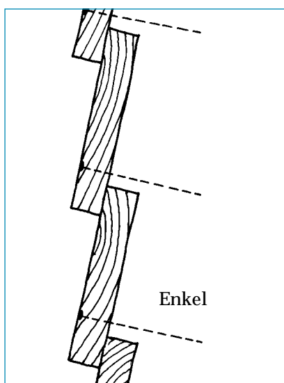
Figur 5. Riktig spikring av liggende kledning.
