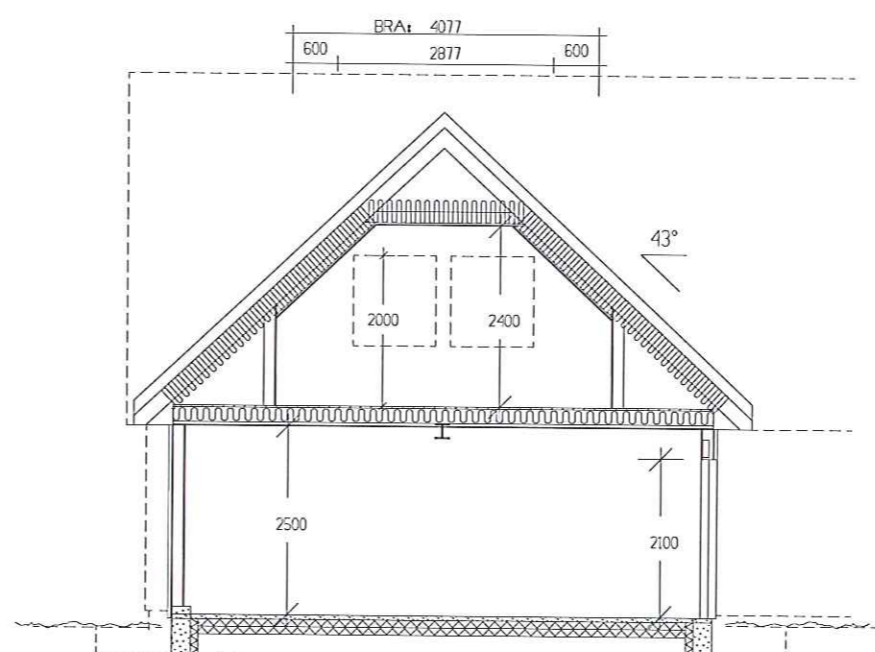
SNITT B-B
