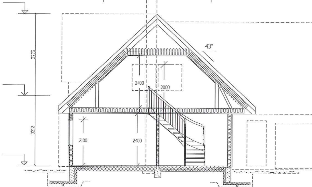
SNITT A-A
