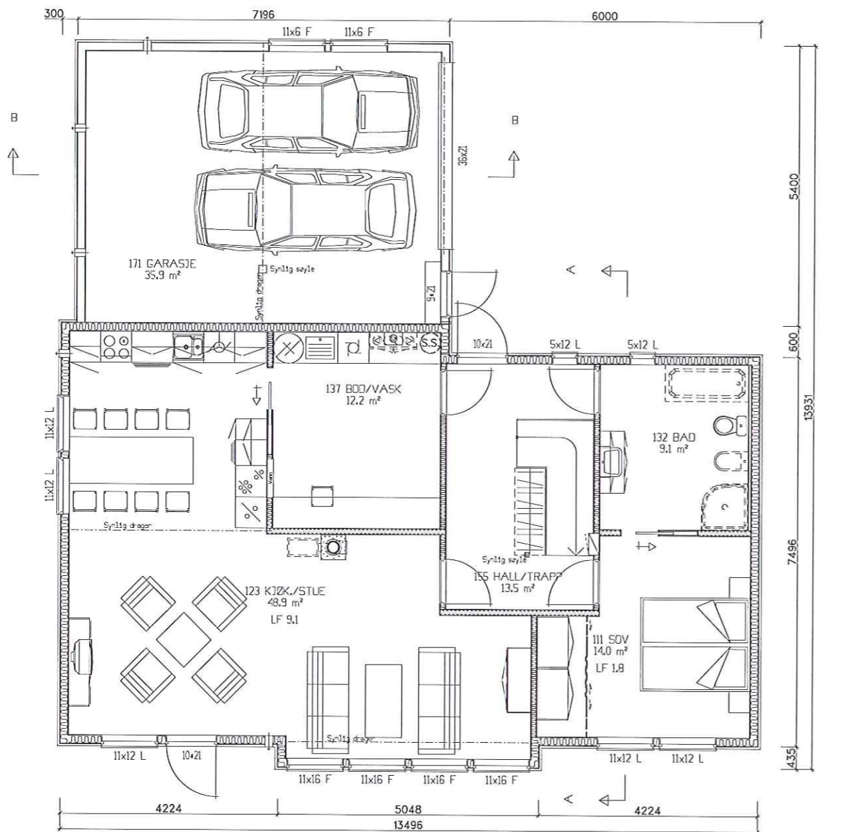
HOVEDPLAN
