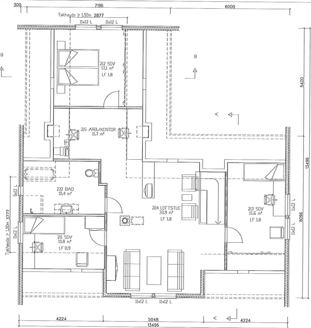
LOFTPLAN
