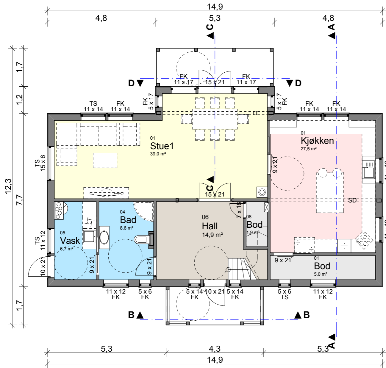
1 ETASJE
