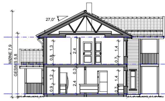
SNITT A-A
