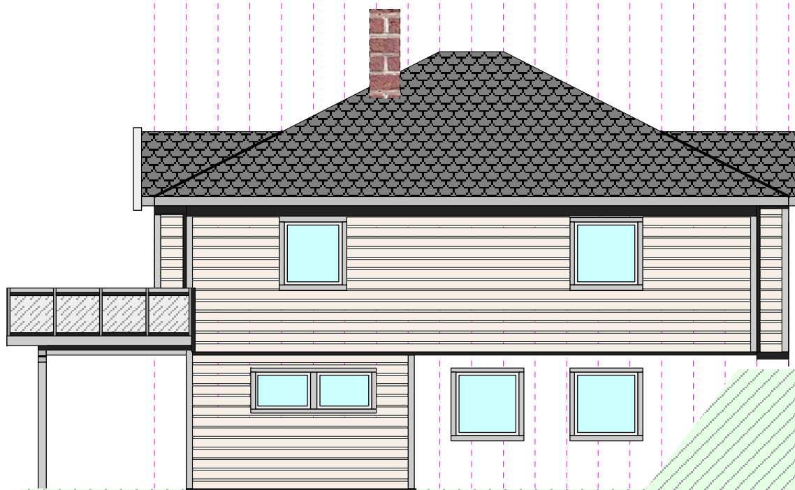
FASADE VEST
