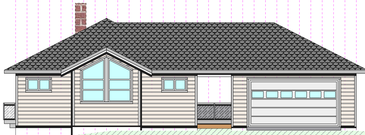
FASADE SØR
