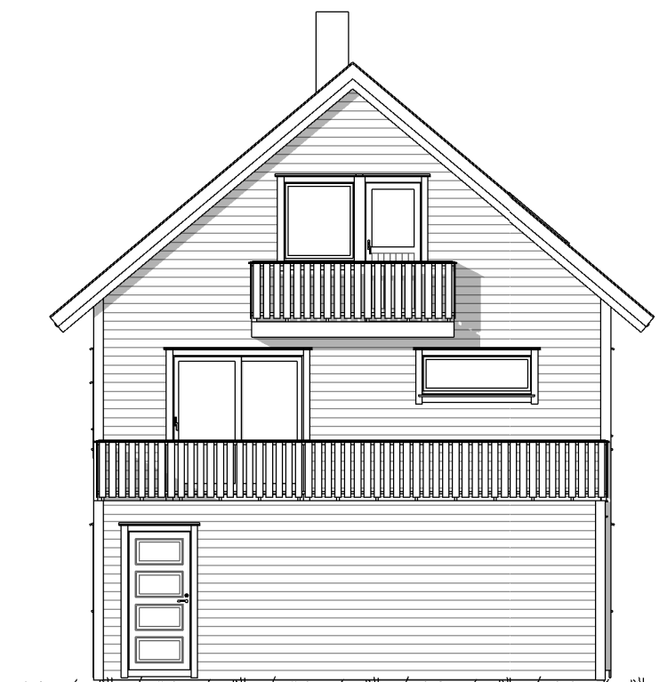
FASADE 4
