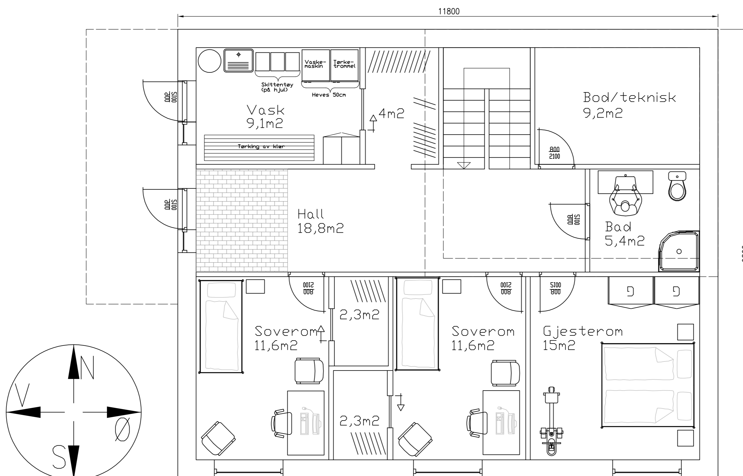
U-etasje
