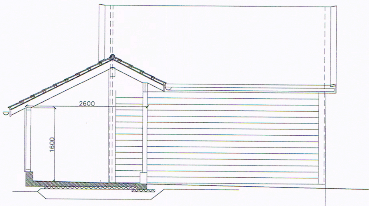
SNITT REDSKAPSHUS
