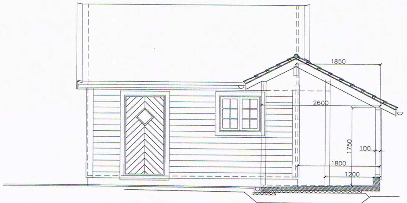
SNITT "GAPAHUET"
