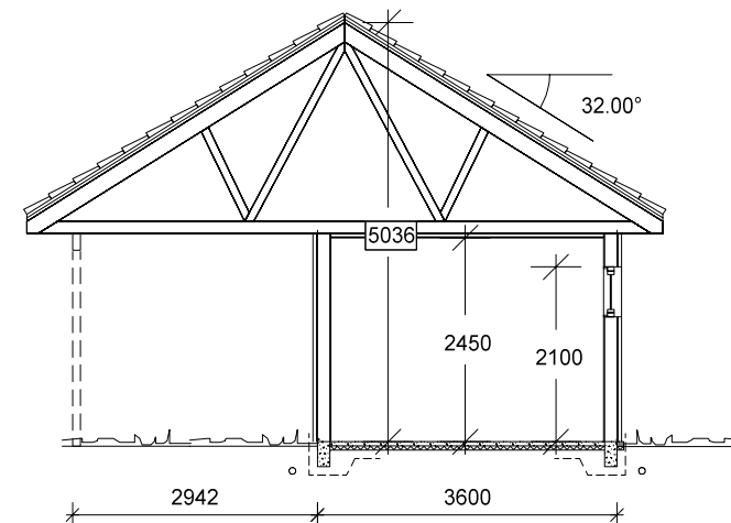
SNITT B-B
