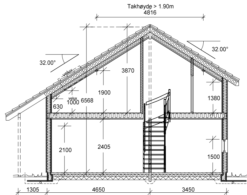
SNITT A-A
