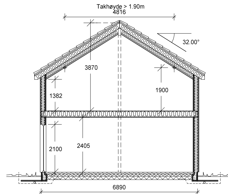
SNITT C-C
