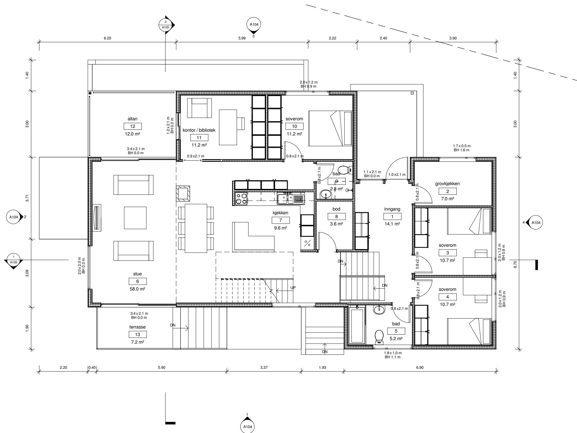
① HOVEDETASJE 1 : 50
