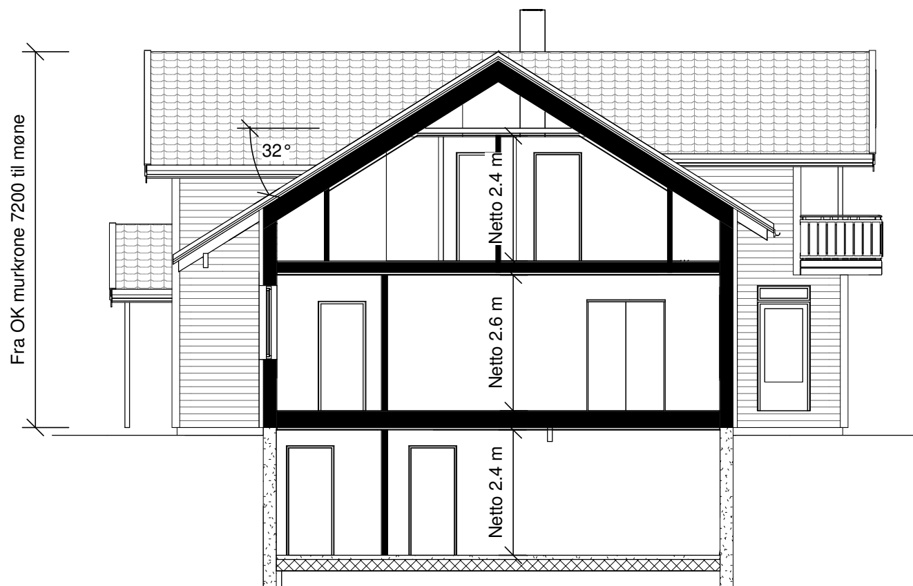
Snitt A - A
