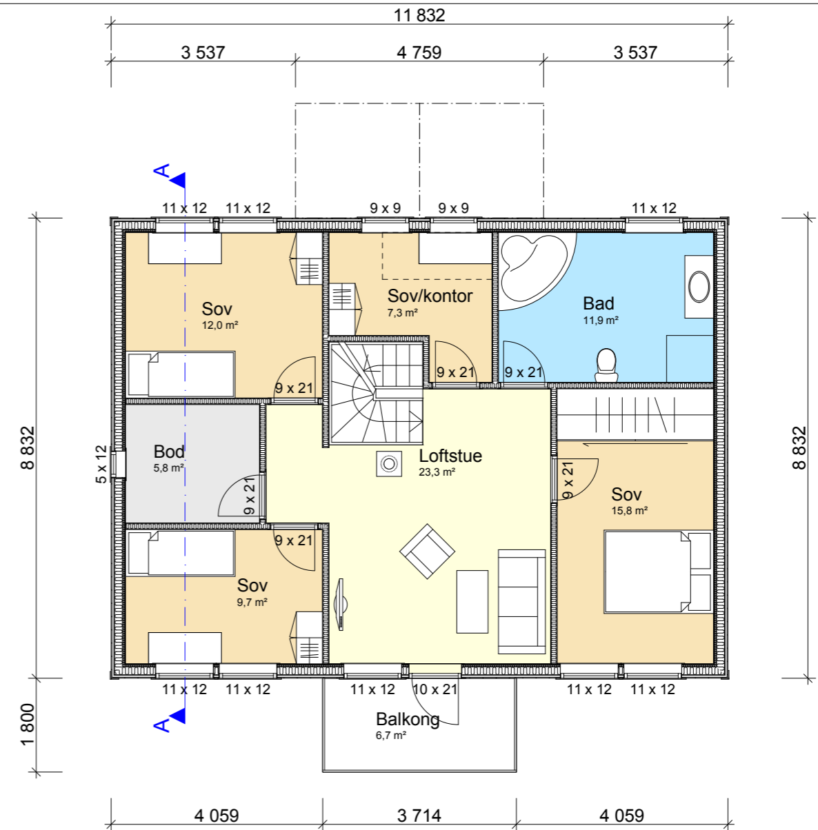
Loftplan 1:100
