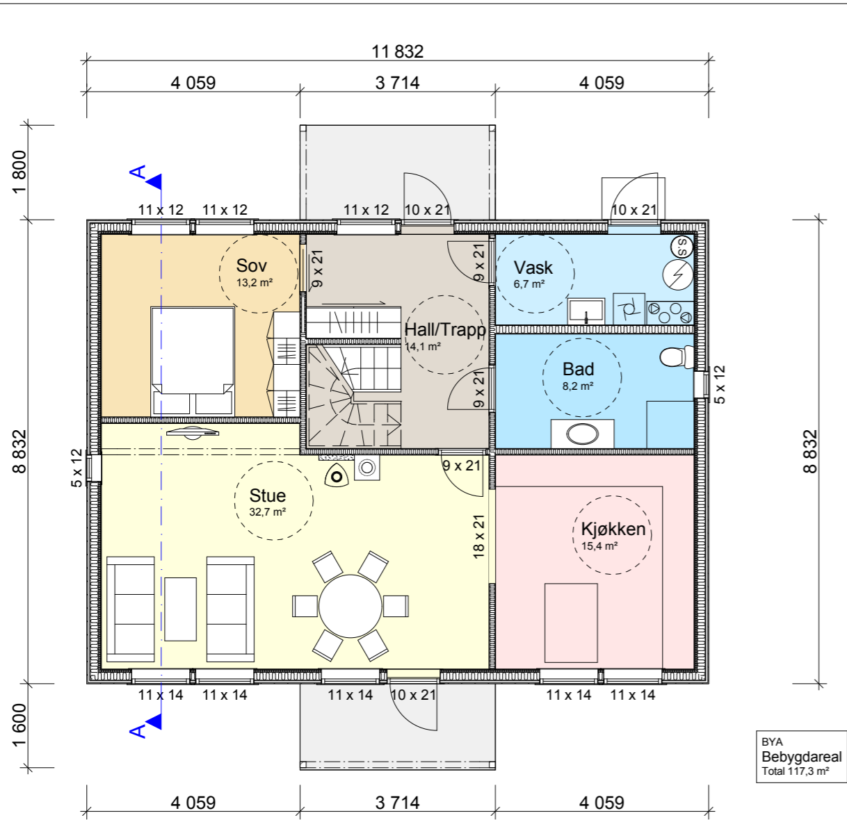
Hovedplan 1:100
