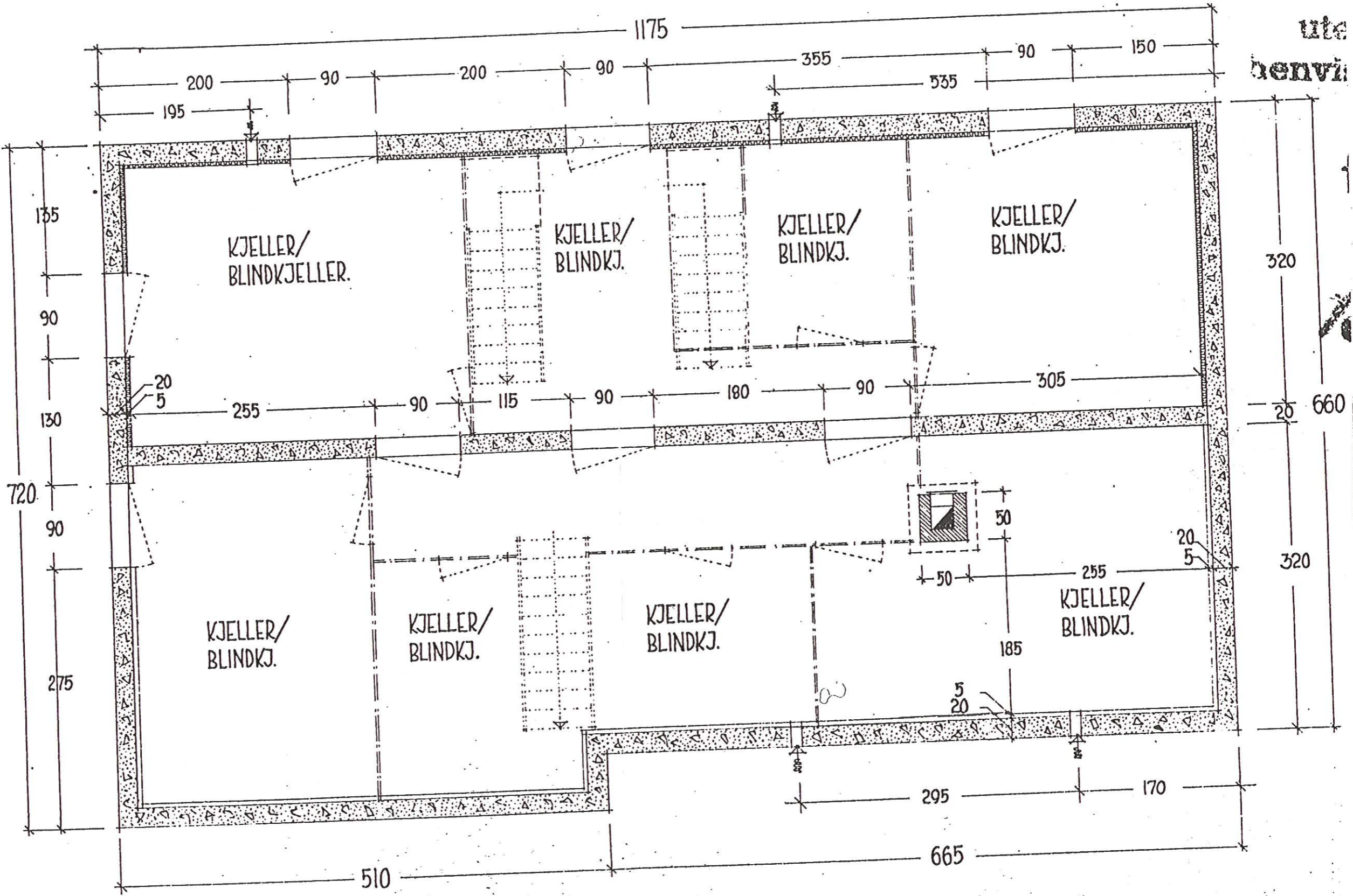
KJELLER-BLINDKJELLER-PLAN.
