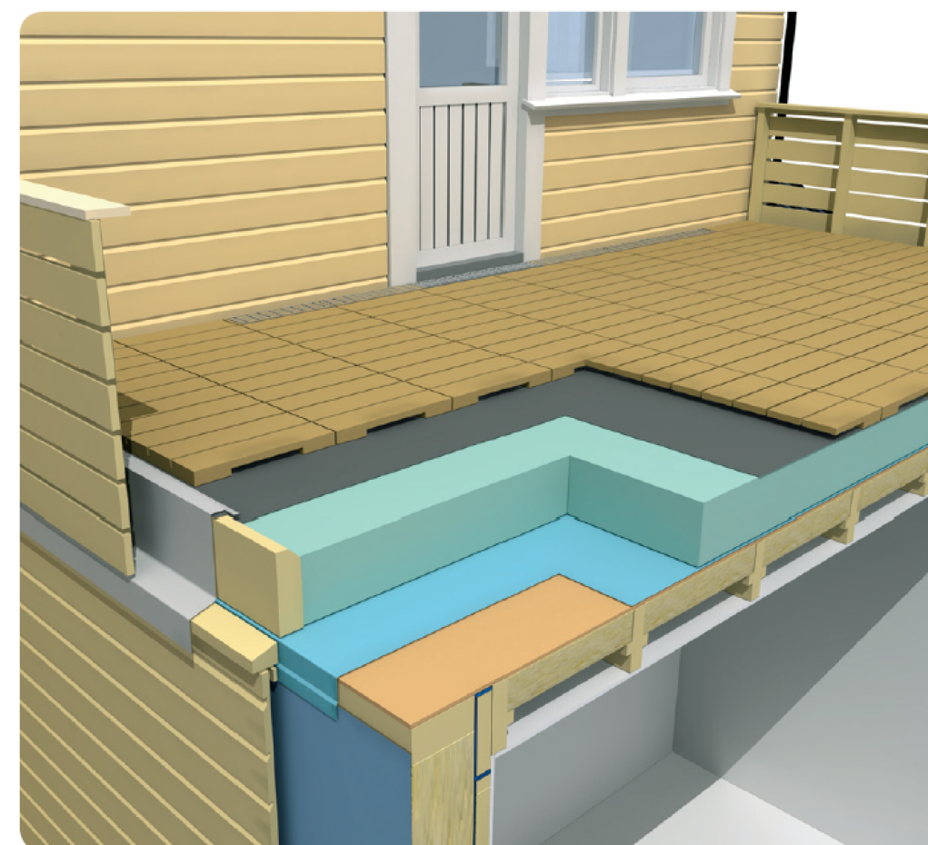
Oppbygging av kompakt tak
