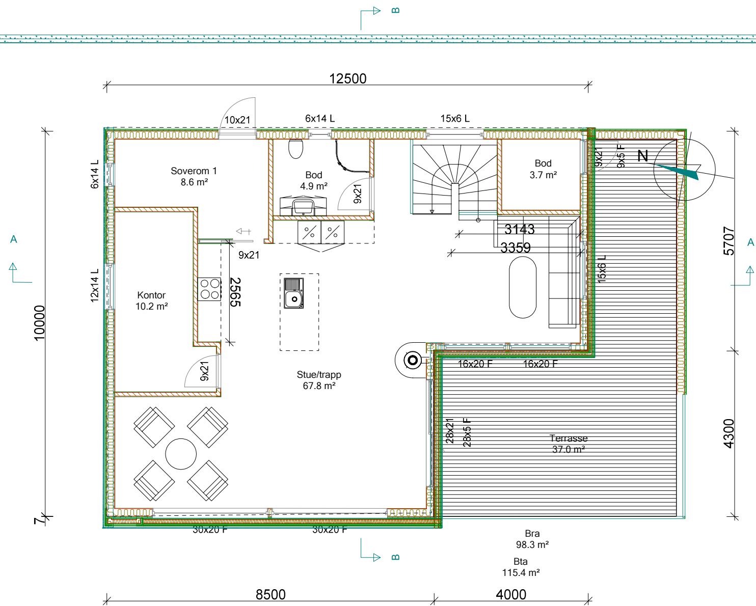
Plantener 1:100 2 etg
