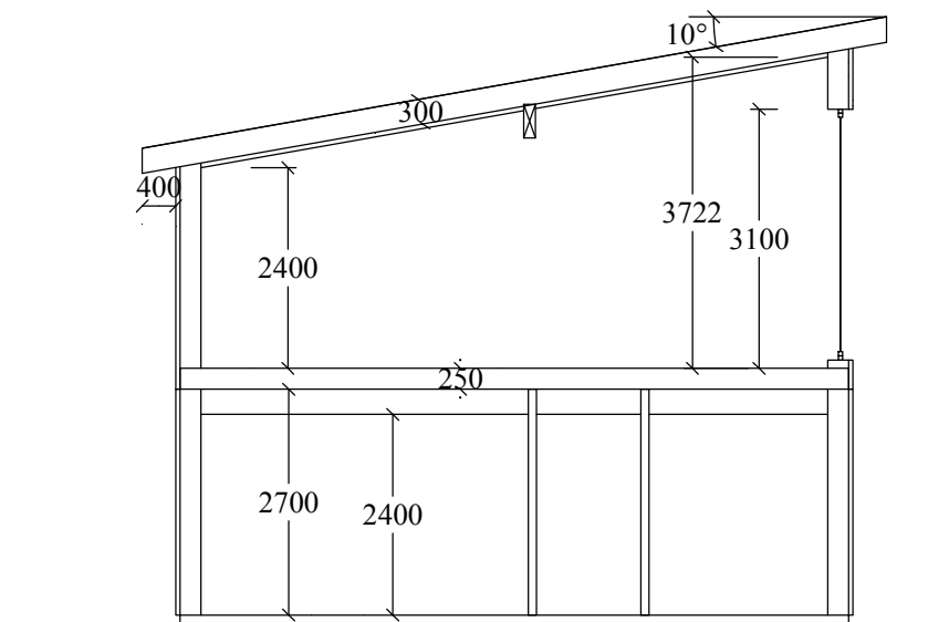
Snitt A-A
