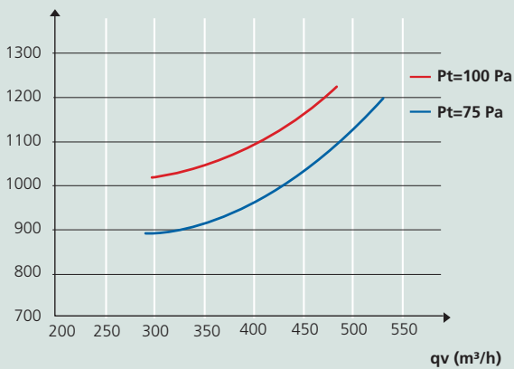
Comfort 450 · SEL (SFP) - kurve · SEL (J/m 3 )
