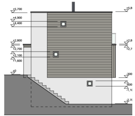
3 Nord høyde 1:1
