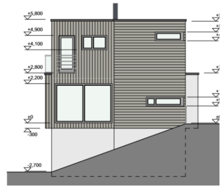
4 Nord høyde 1:1
