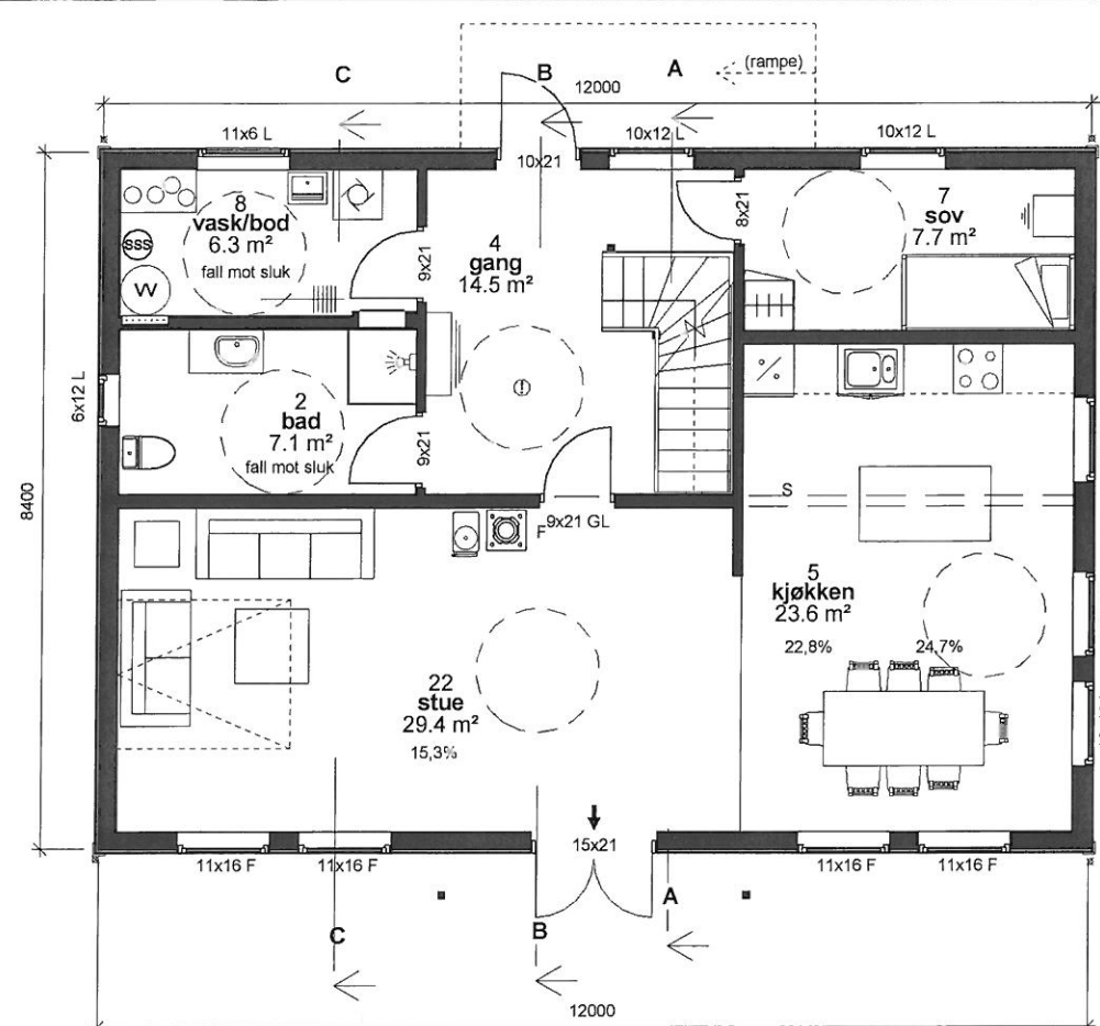
2.0 Hovedetasje 1 : 100
