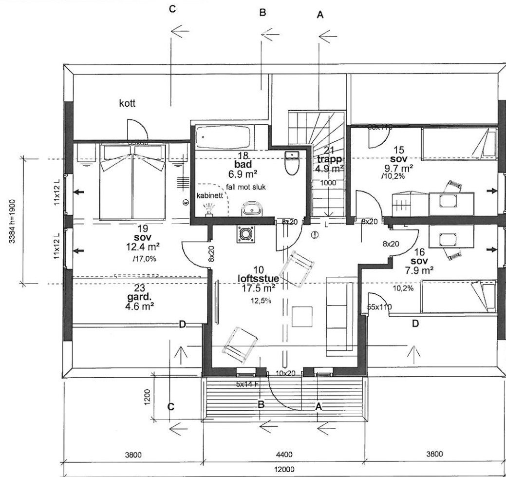
3.0 Loftsetasje 1 : 100
