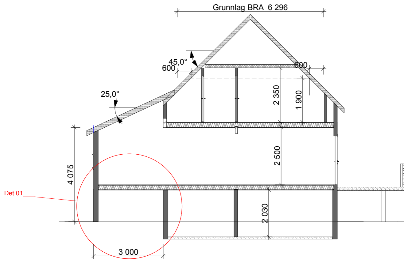
1:100 Snitt B
