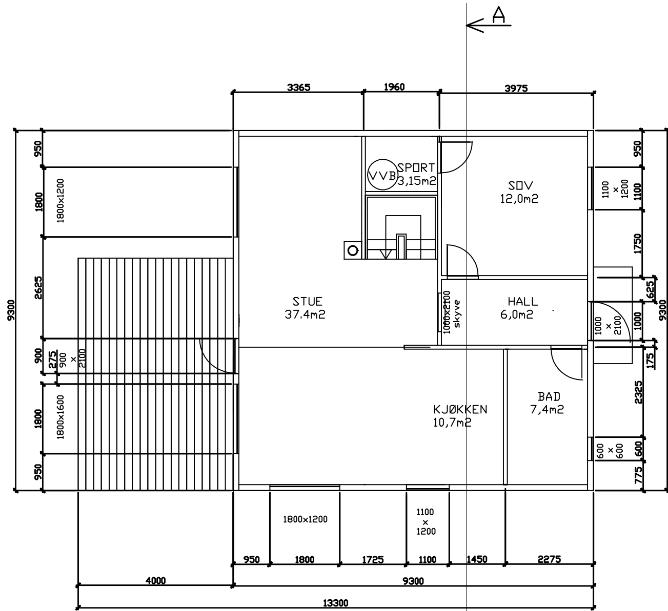
Grunnplan 1. etasje
