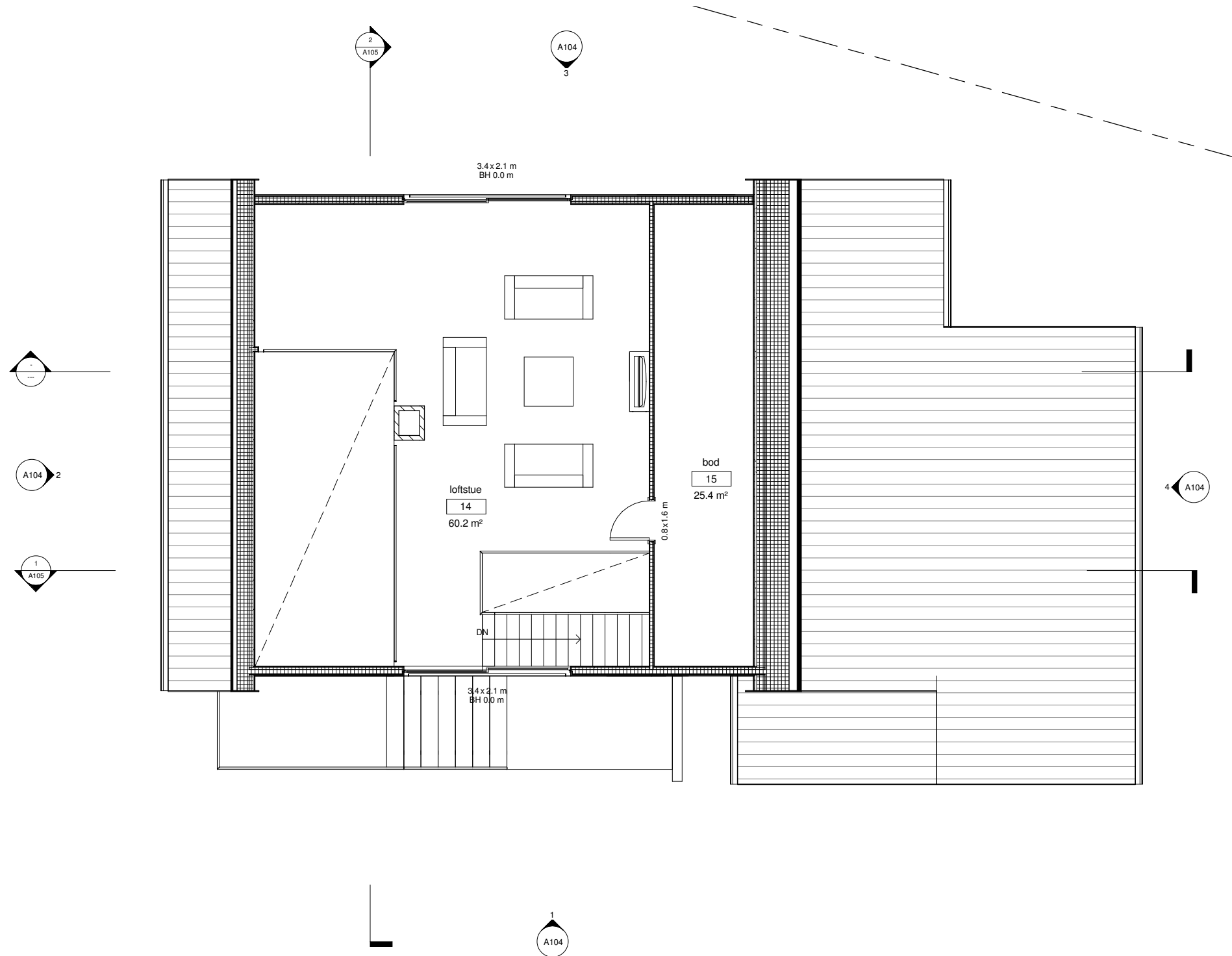
① LOFTETASJE 1 : 50
