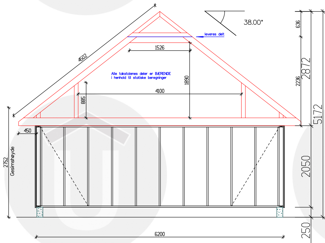
Snitt - 1:50
