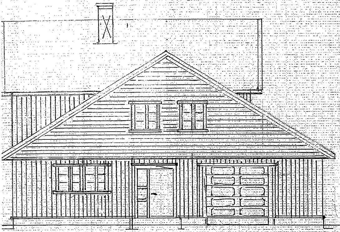
Fasade Nord
