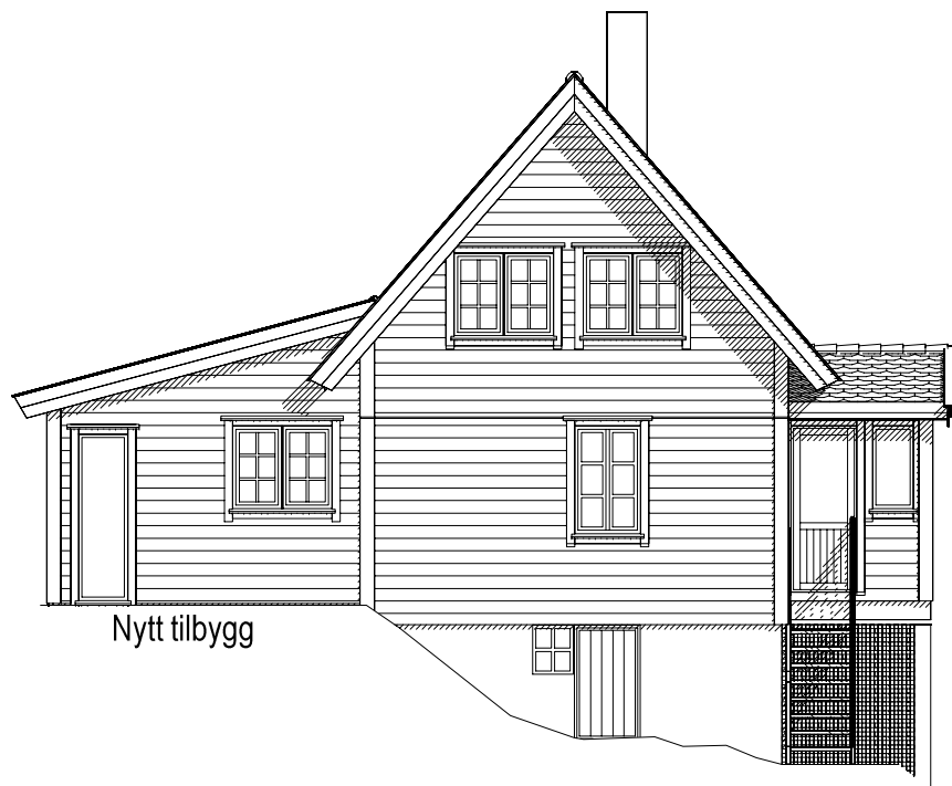
FASADE MOT ØST
