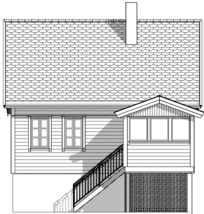
FASADE MOT NORD Nytt: Vinduer ved inngangsparti
