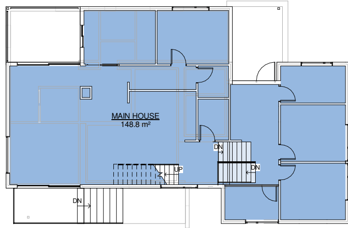
③ HOVEDETASJE 1 : 100
