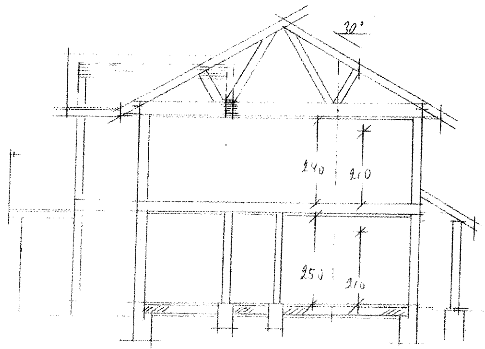
SNITT
