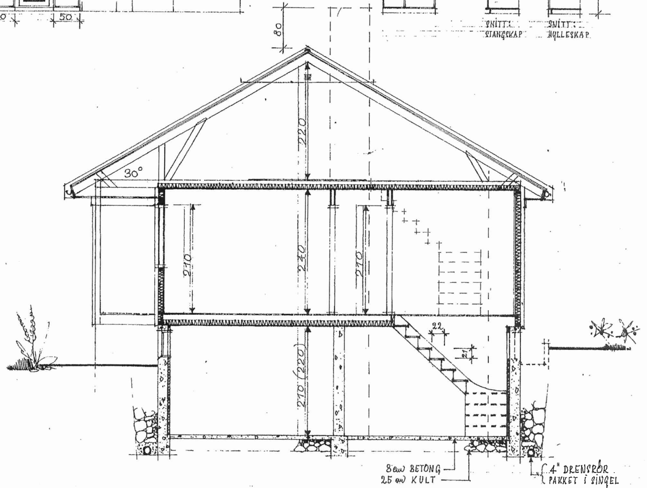
SNITT A-A
