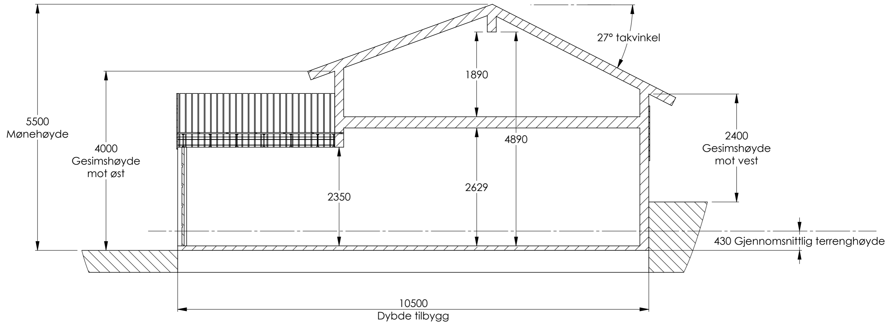
SNITT A-A (sett fra eksisterende bygning/nord Målestokk 1:50
