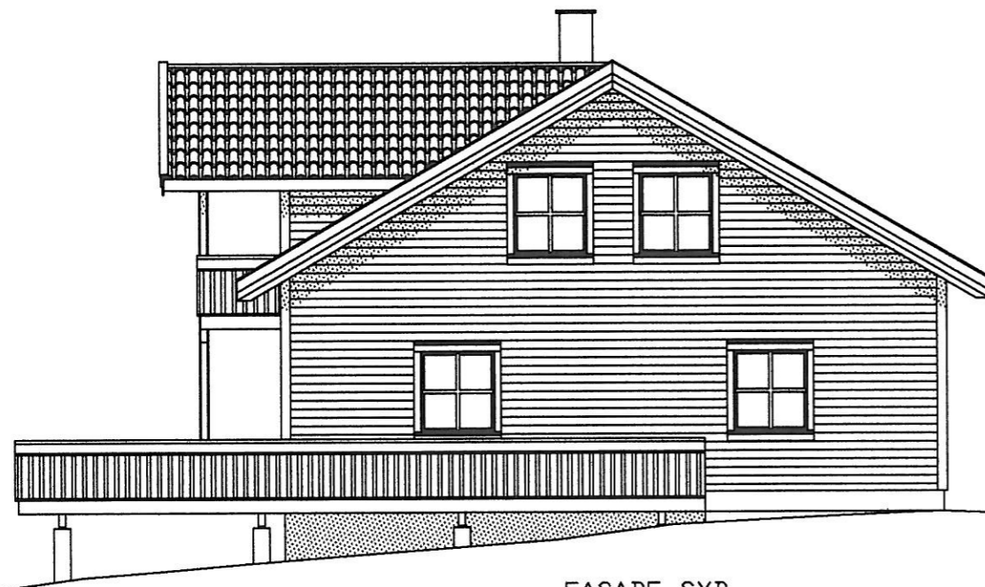
FASADE SYD
