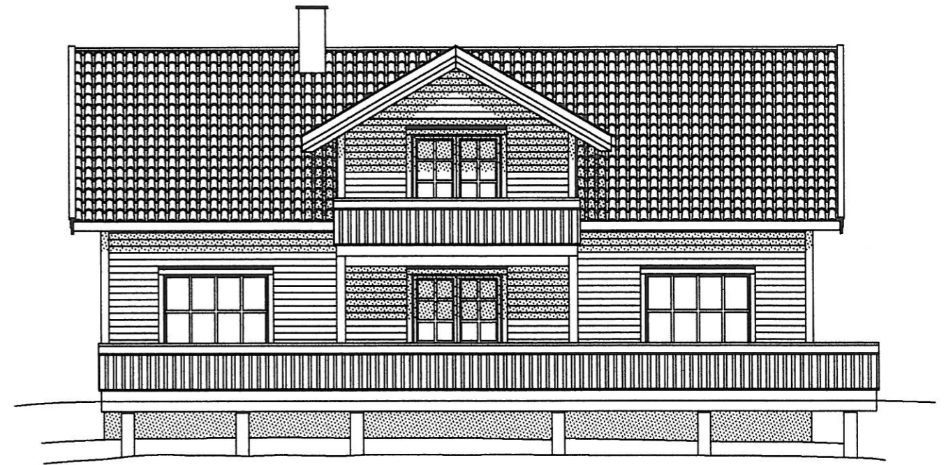
FASADE VEST
