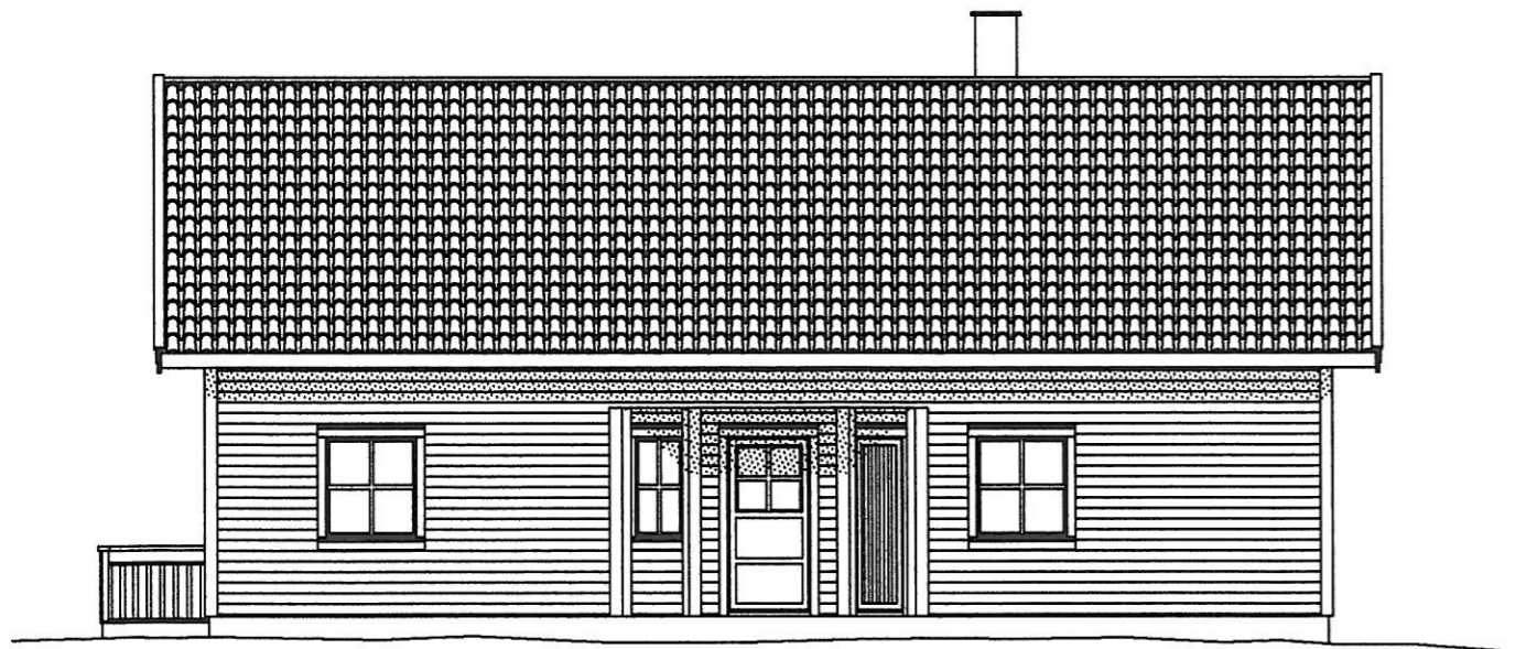
FASADE ØST
