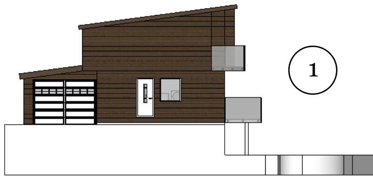
Fasade nordvest
