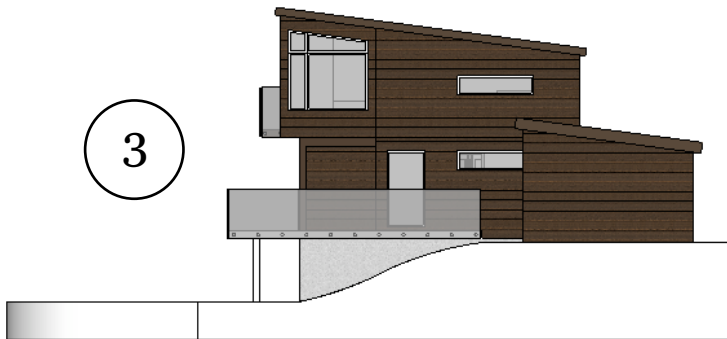
Fasade sørøst
