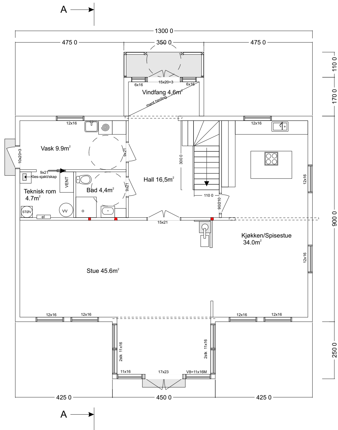
Plan 1etg
