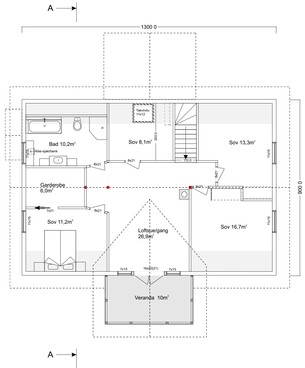
Plan 2etg
