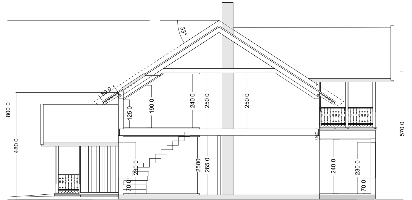
Snitt
