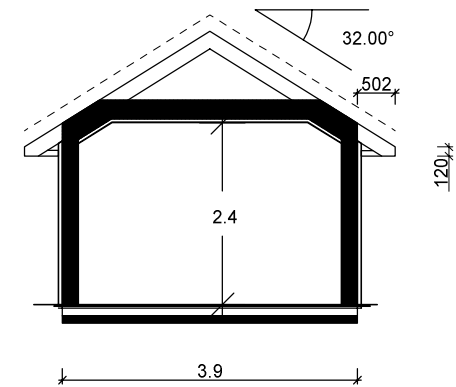
Snitt B-B
