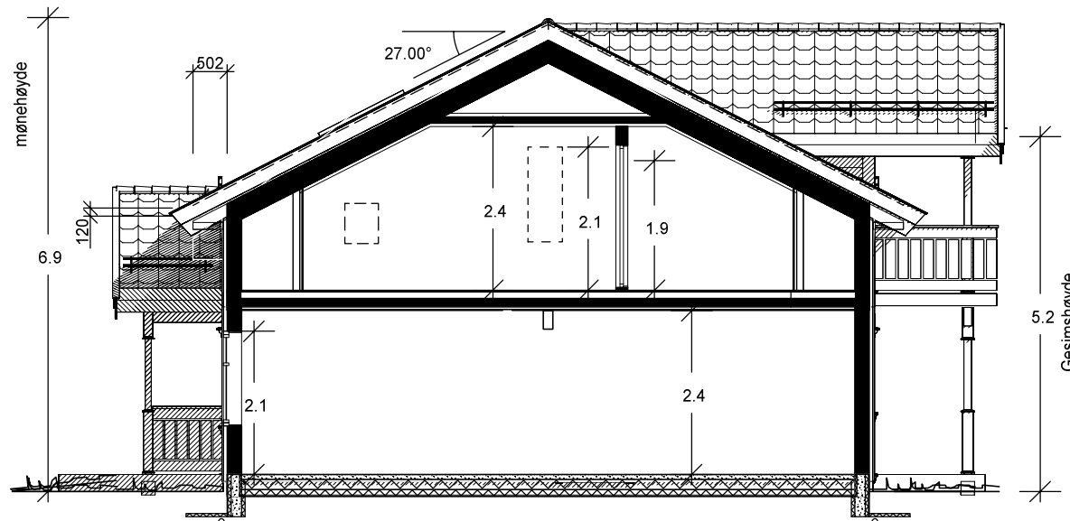
Snitt A-A
