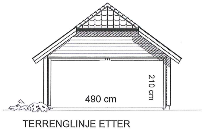
FASADE NORD
