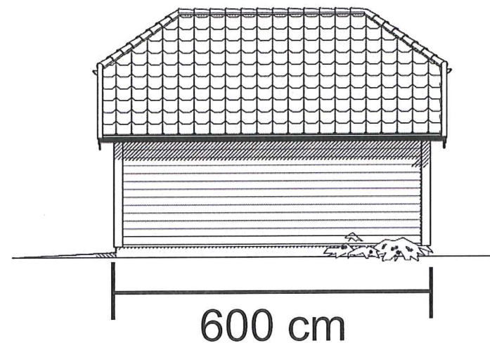
FASADE VEST
