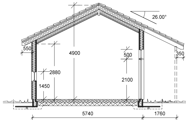
SNITT D-D
