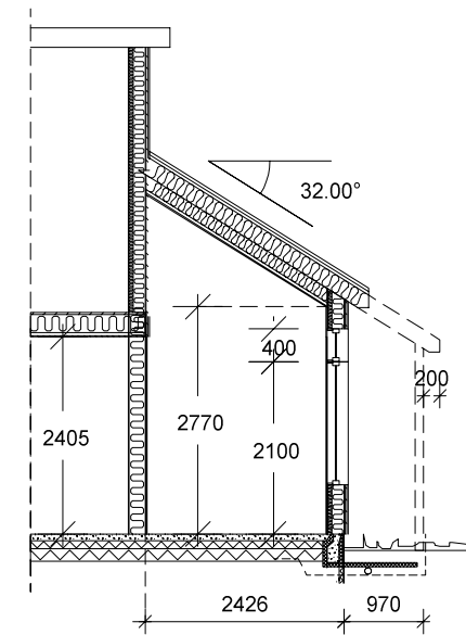
SNITT E-E
