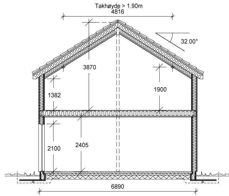
SNITT C-C
