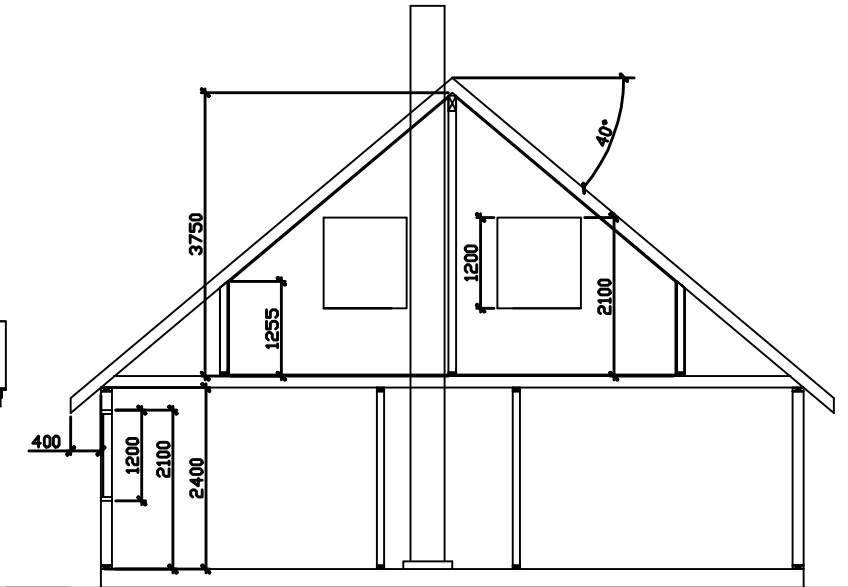
SNITT A-A
